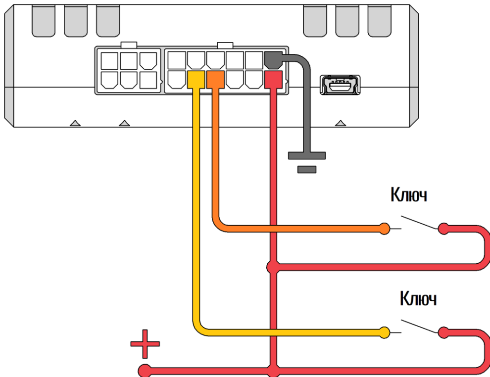
Рисунок 2.14 Подключение с подтяжкой к «-»
