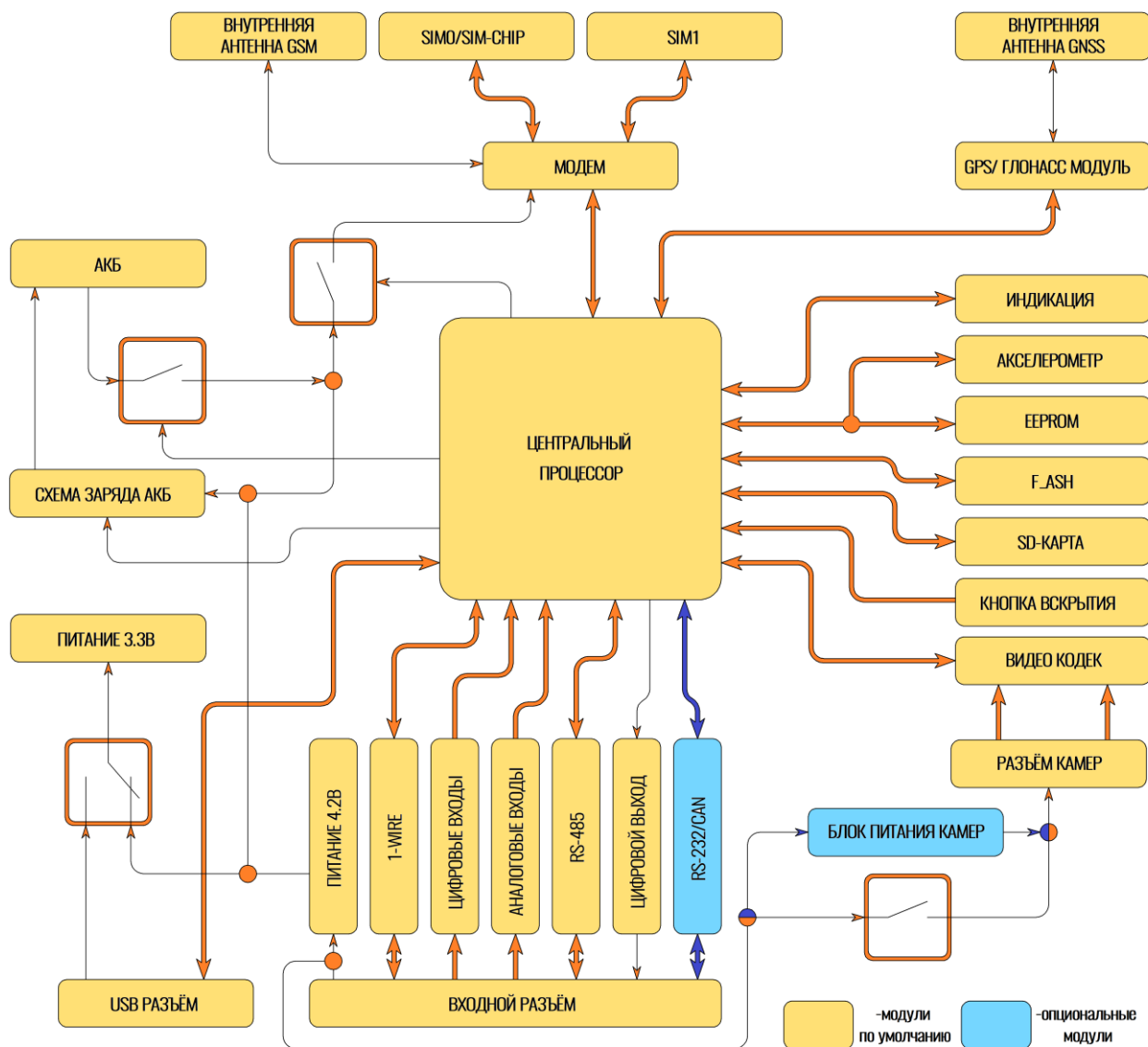
Рисунок 1.3 Блок-схема навигационного терминала
