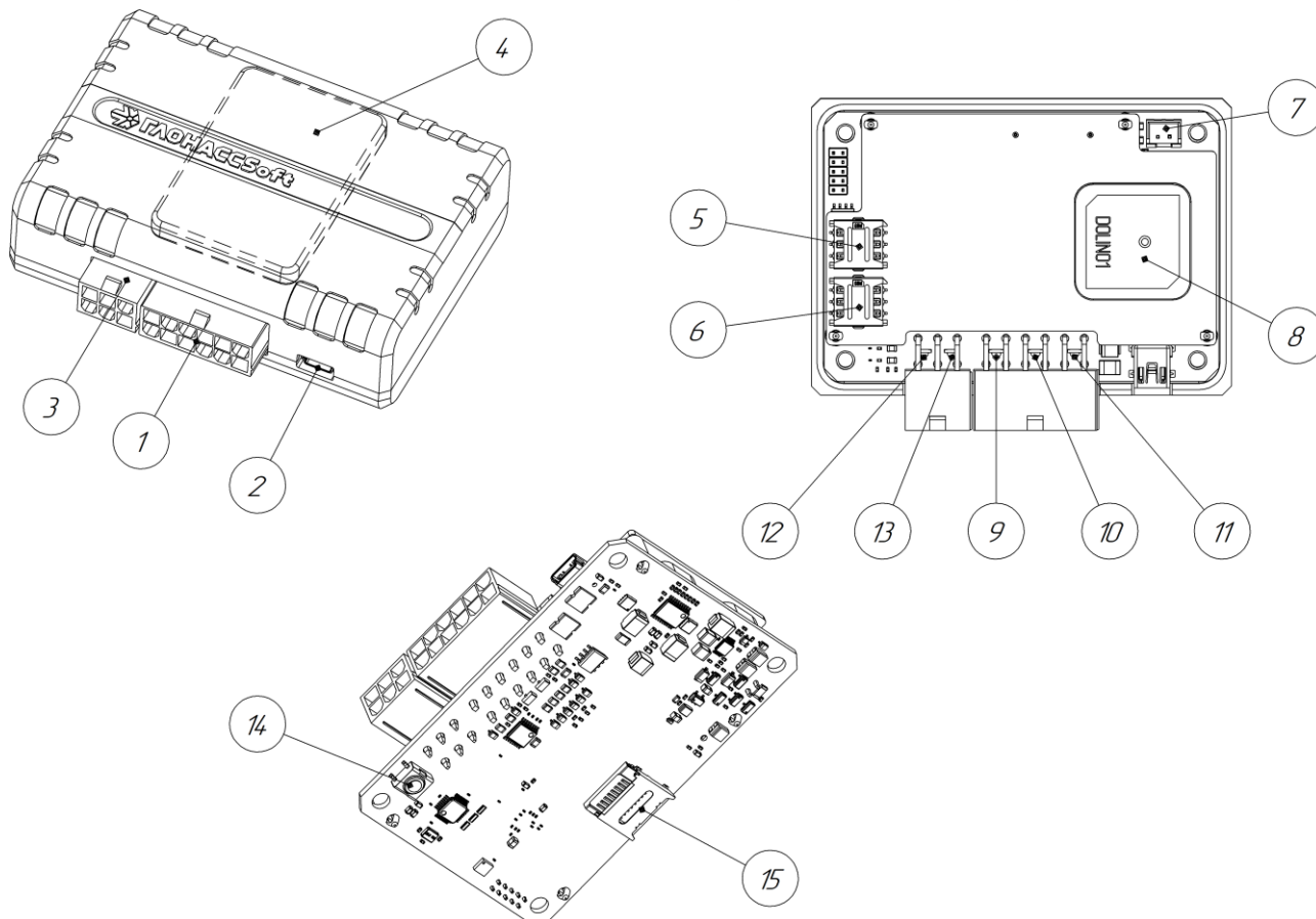
Рисунок 2.5 Основные элементы терминала
