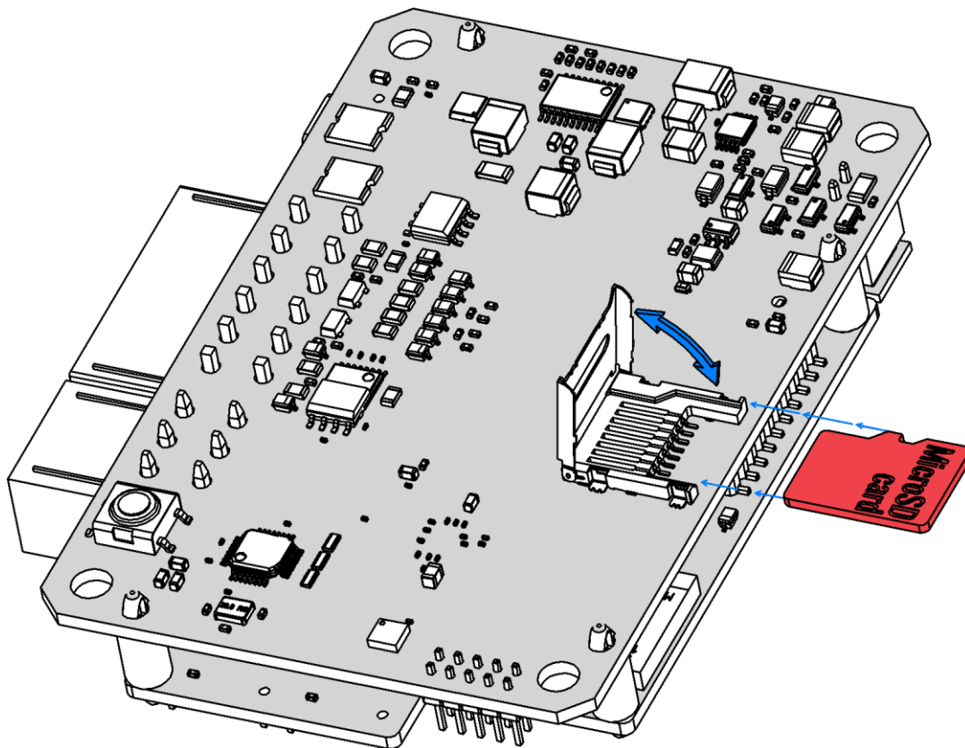
Рисунок 2.10 Установка microSD-карты
